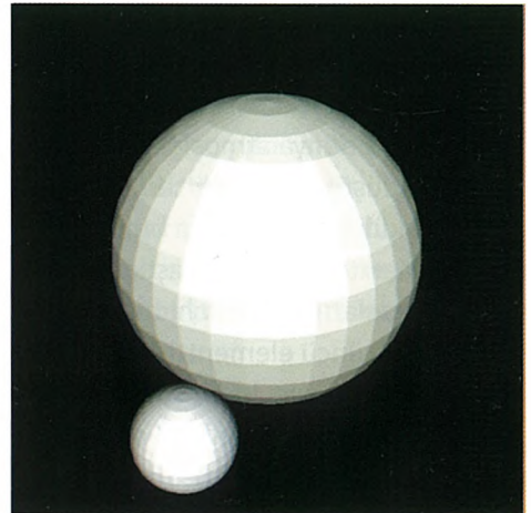
Resim 1: Hidrojen molekülü
